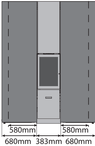
SYMÉTRIQUE LARGE
