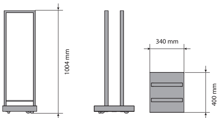
CHARIOT À BÛCHES
